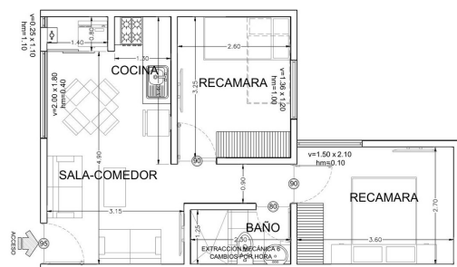
1 DEPARTAMENTOS TIPO F1 AREA= 45.92 M2 DEP. B-002
